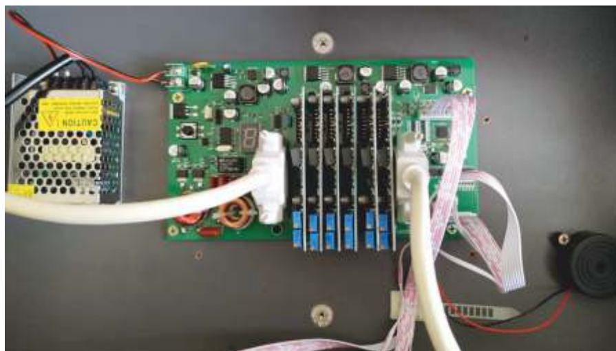
Рисунок 4. Материнская плата.
