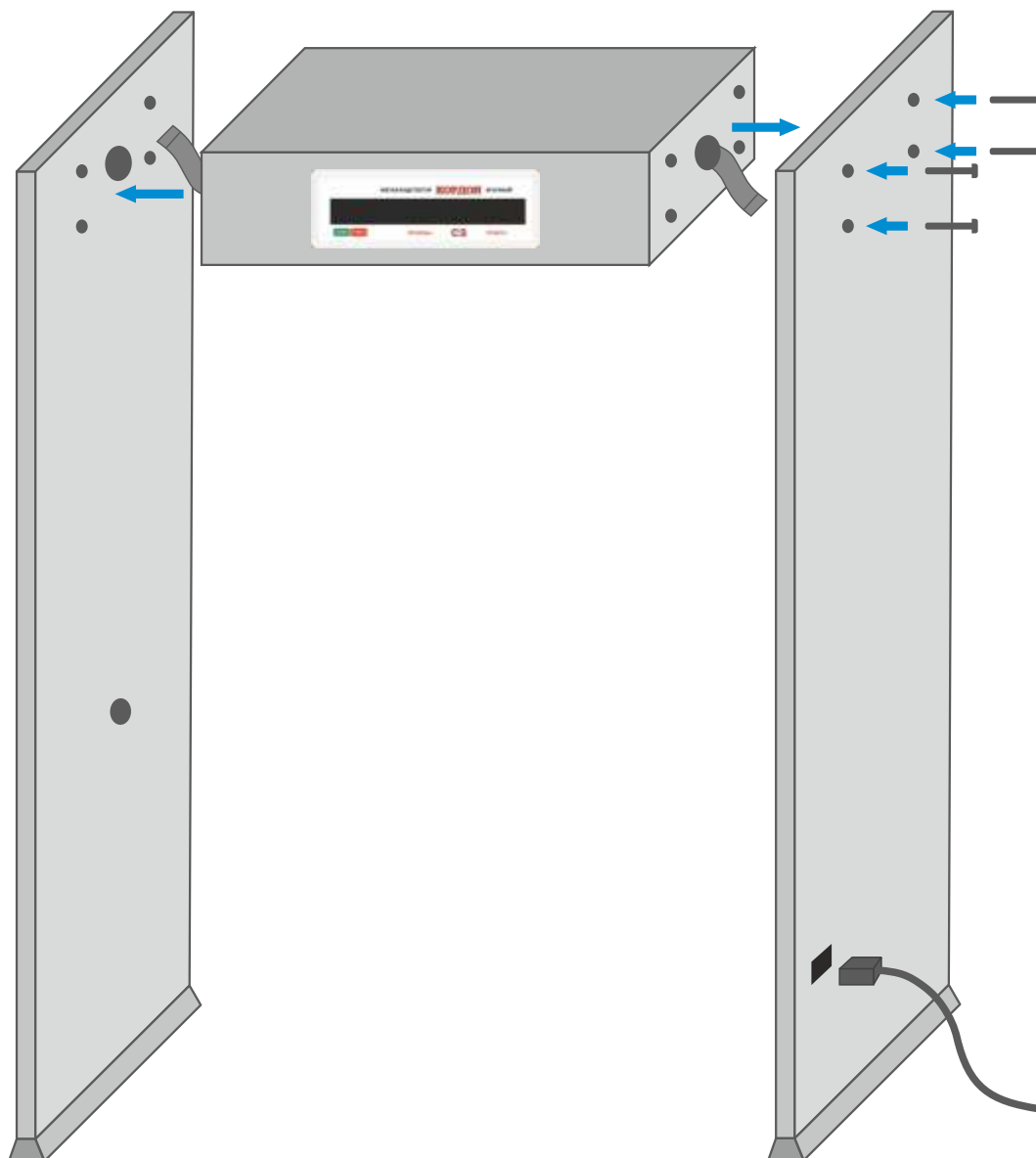
Рисунок 3. Сборка металлодетектора.
